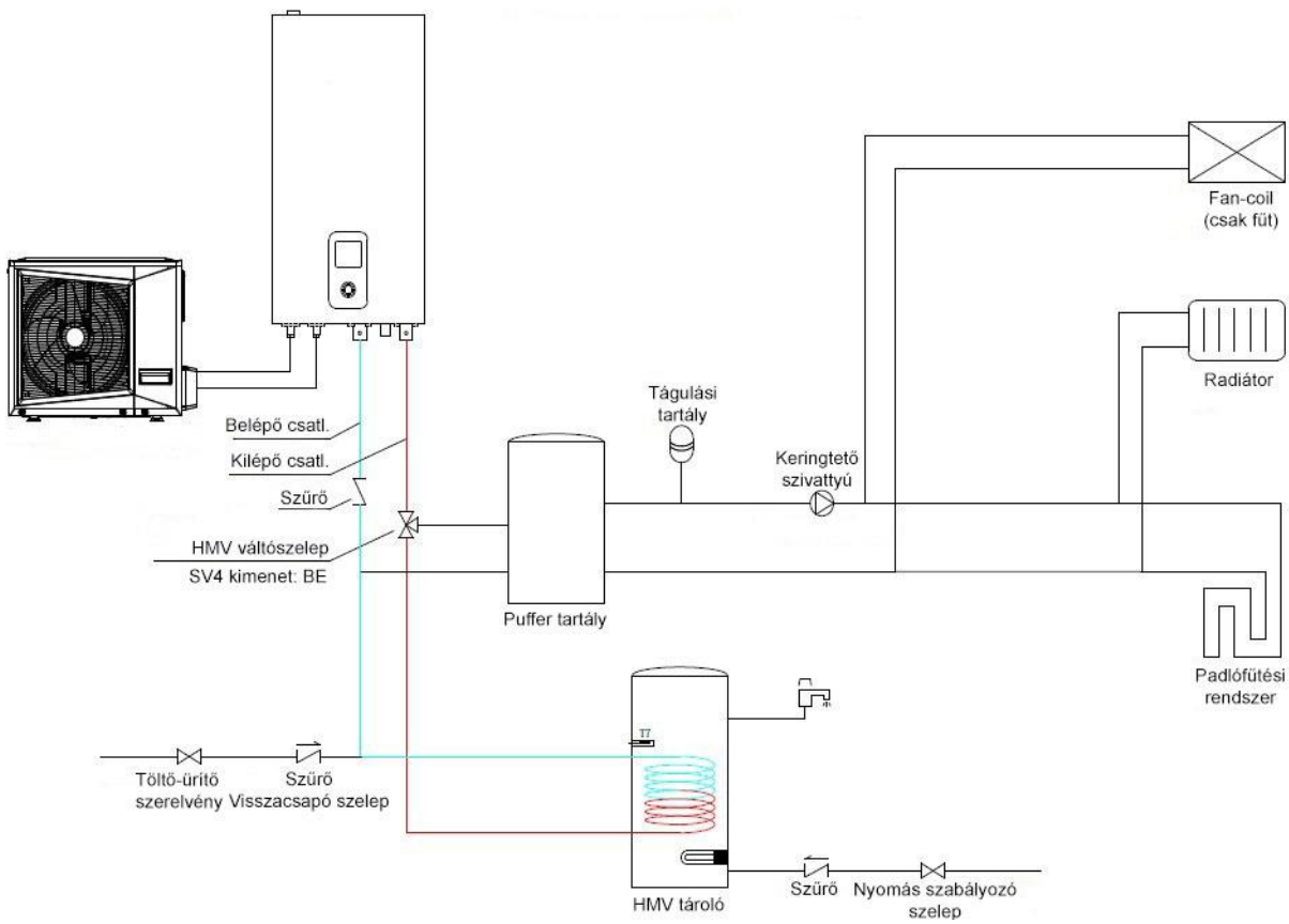
Fűtés és használati melegvíz előállítás – HMV üzemmódban
