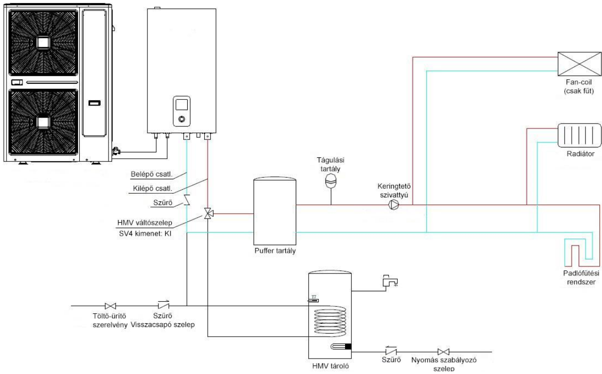
Fűtés és használati melegvíz előállítás – Fűtés üzemmódban
