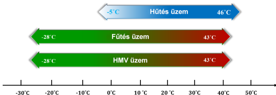
3-2. kép: Működési hőmérséklet-tartomány
