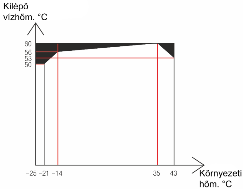
4-3. kép: A használati melegvízes üzemmód működési tartománya
