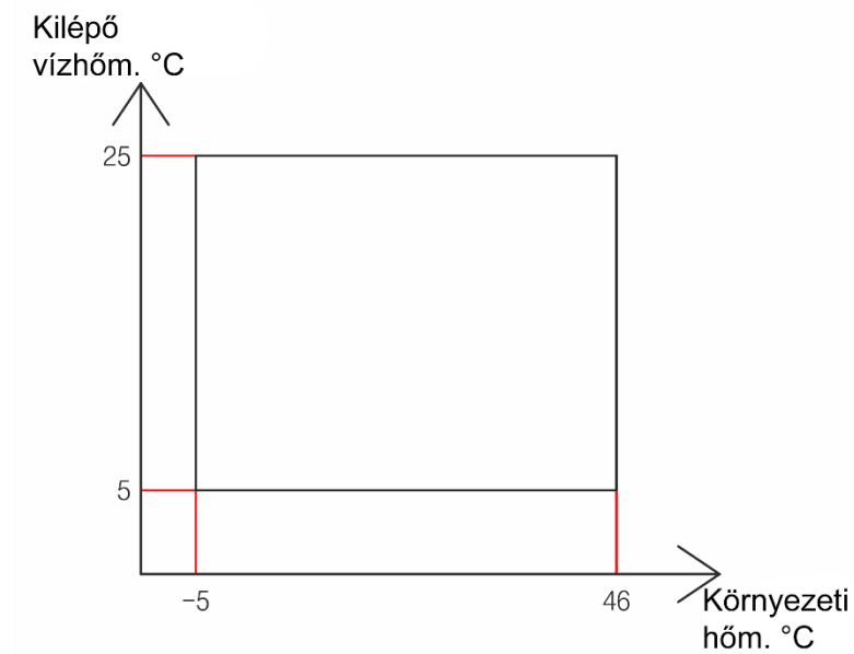
4-2. kép: A hűtési üzemmód működési tartománya
