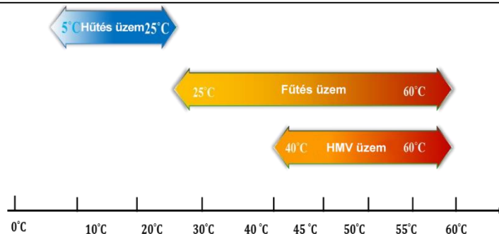
3-3. kép: Kilépő vízhőmérséklet tartomány
