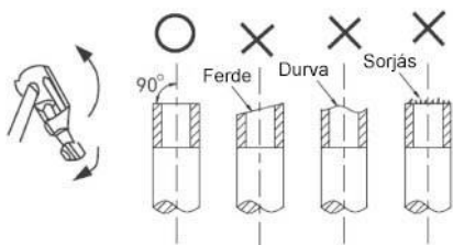
A cső vágása
