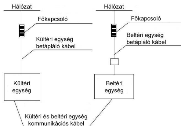
Vezetékezés és vezérlés
