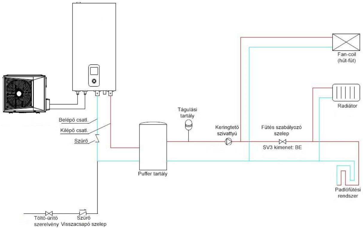
Hűtés és fűtés, HMV előállítás nélkül – Fűtés üzemmódban
