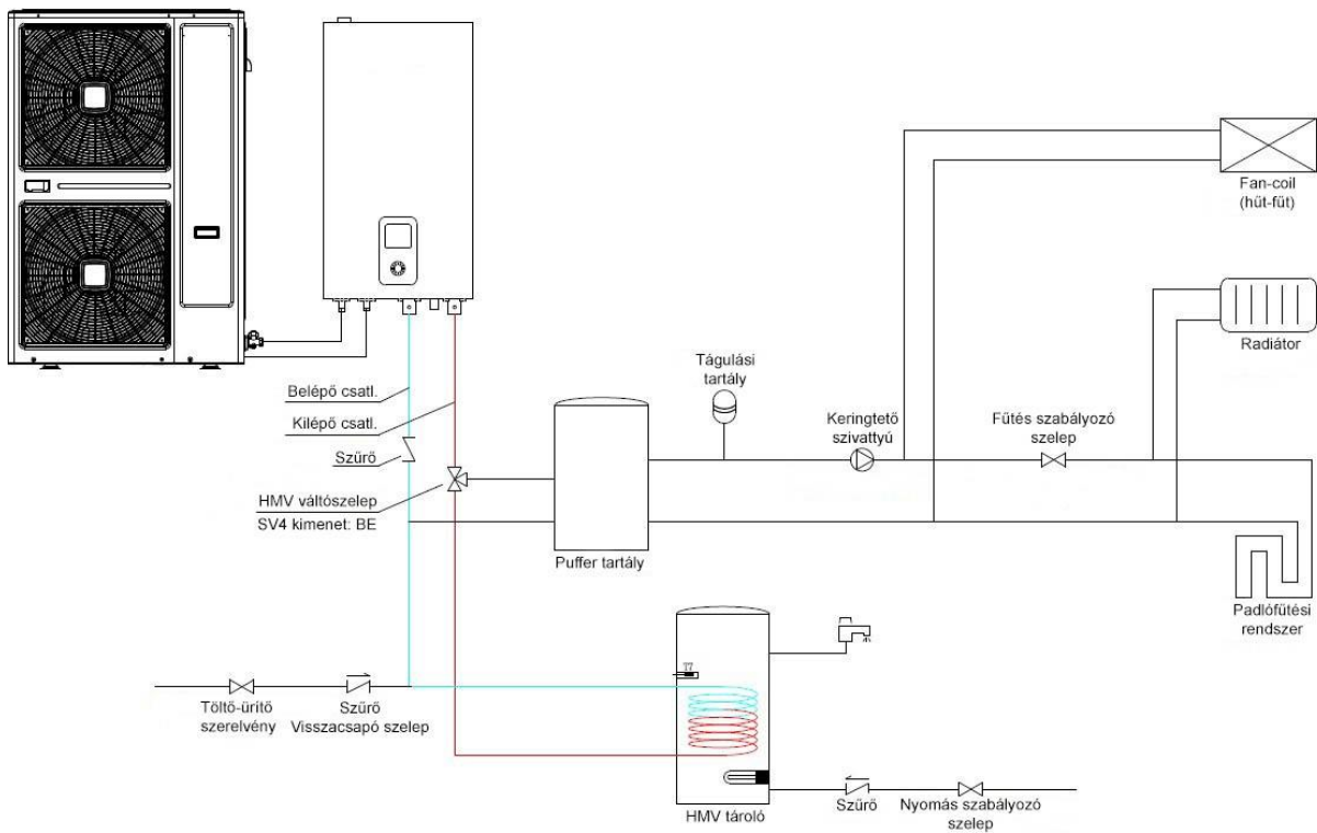
Hűtés, fűtés és használati melegvíz előállítás – HMV üzemmódban
