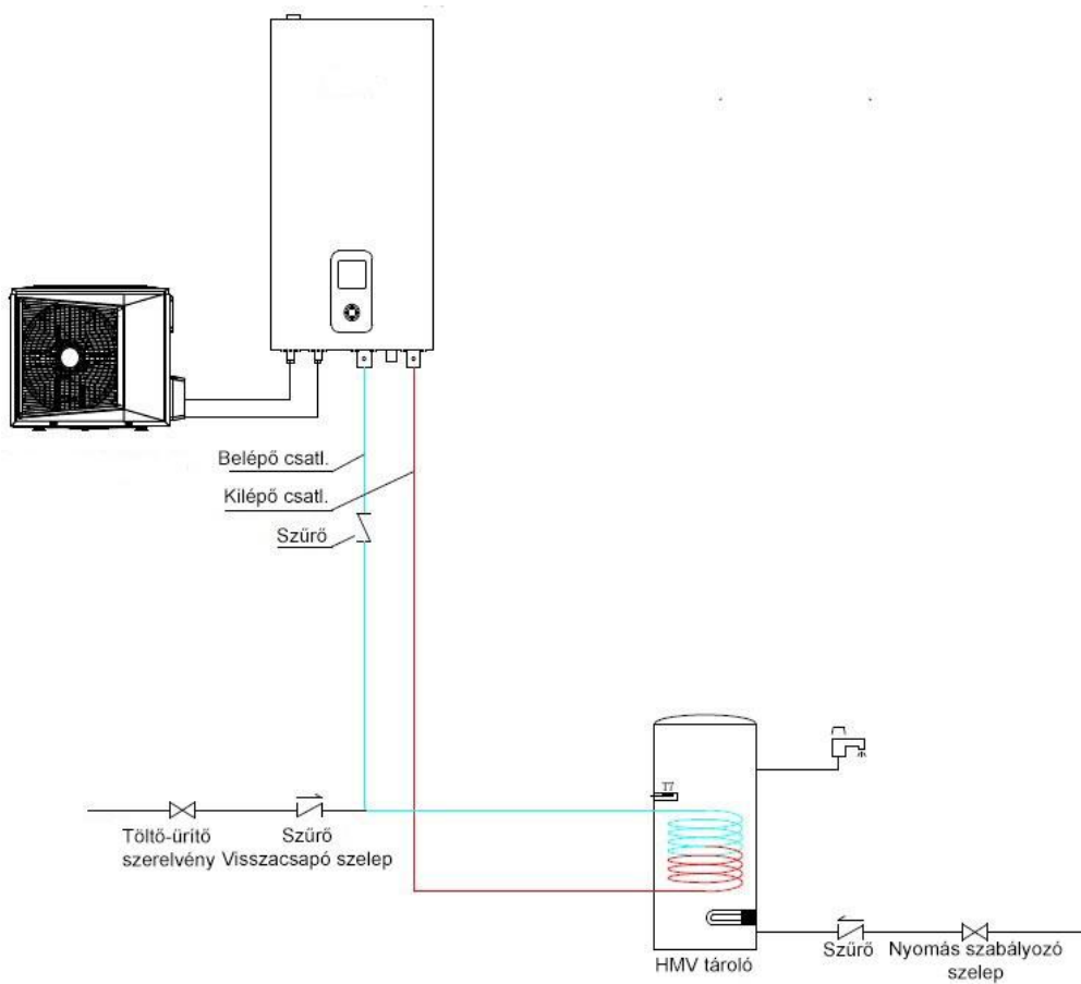
Csak használati melegvíz előállítás
